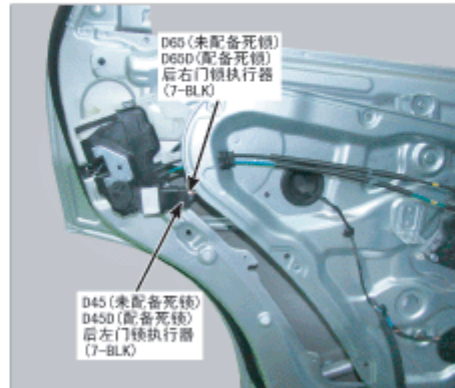
107. 后车门模块
