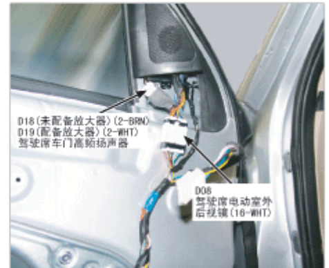
108. 驾驶席车门
