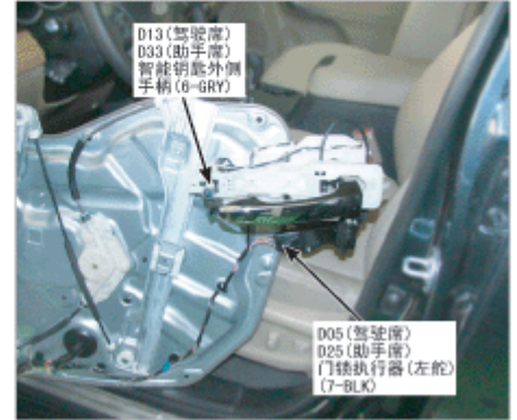
105. 前车门模块
