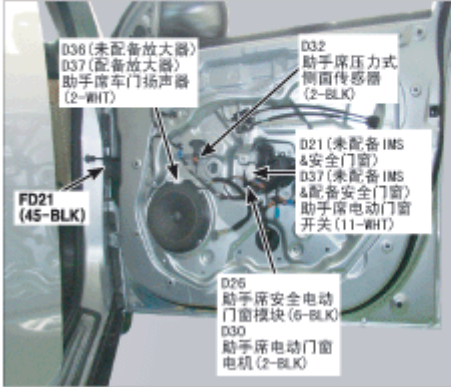
103. 助手席车门
